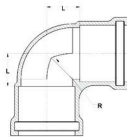
90 Bend
